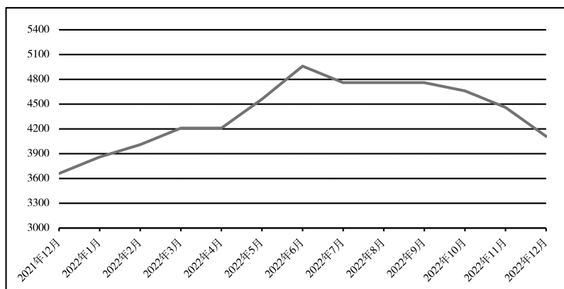
重交道路沥青(AH-70)价格走势（元/吨）
